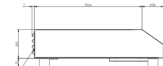
Oldalnézet
